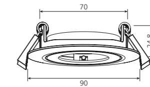
TILT TRIM Ø80
