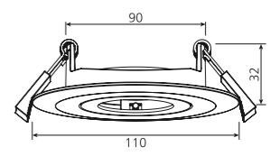
TILT TRIM Ø95
